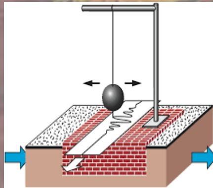
сейсмограф
